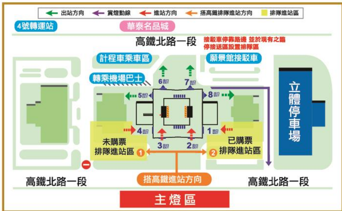
燈會期間高鐵桃園站進出動線及配置示意圖
